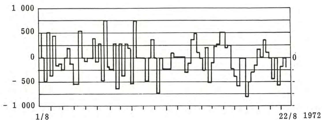
Figur 5 Vattentransporter beräknade från termoklinens vertikala variationer 1972, 1973 och 1974
