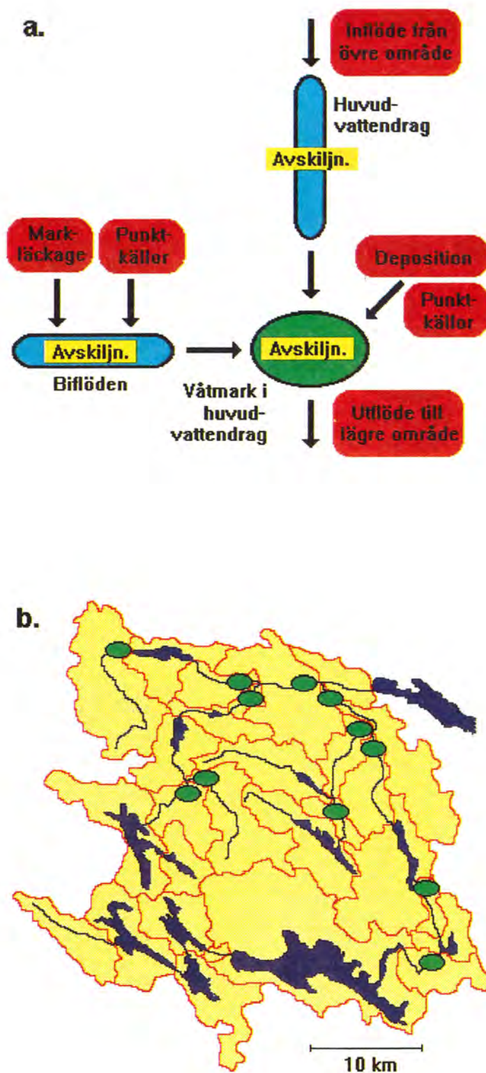
Figur 6. Schematisk beskrivning av modellens kväverutin med hypotetiska våtmarker anlagda i huvudåfåran (a), samt lokaliseringen av dessa i Söderköpingsåns avrinningsområde (b).
