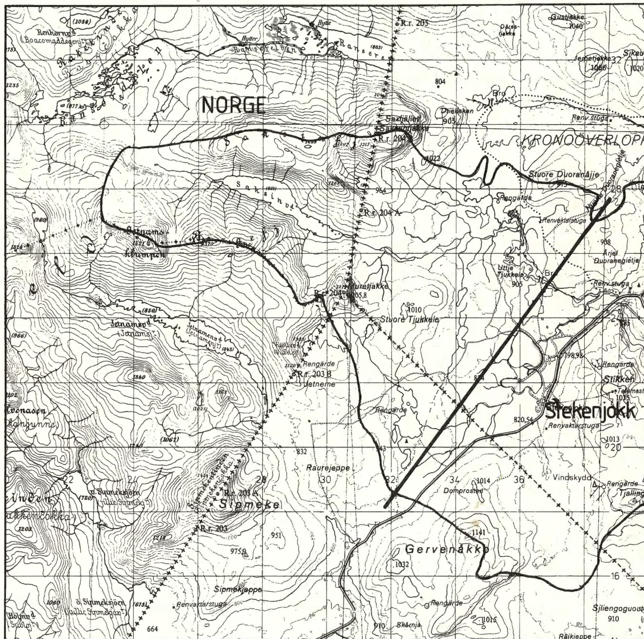
Figur 1. Den västra delen av Kultsjöns avrinningsområde, för vilken snötäckningsgraden bestämts.
