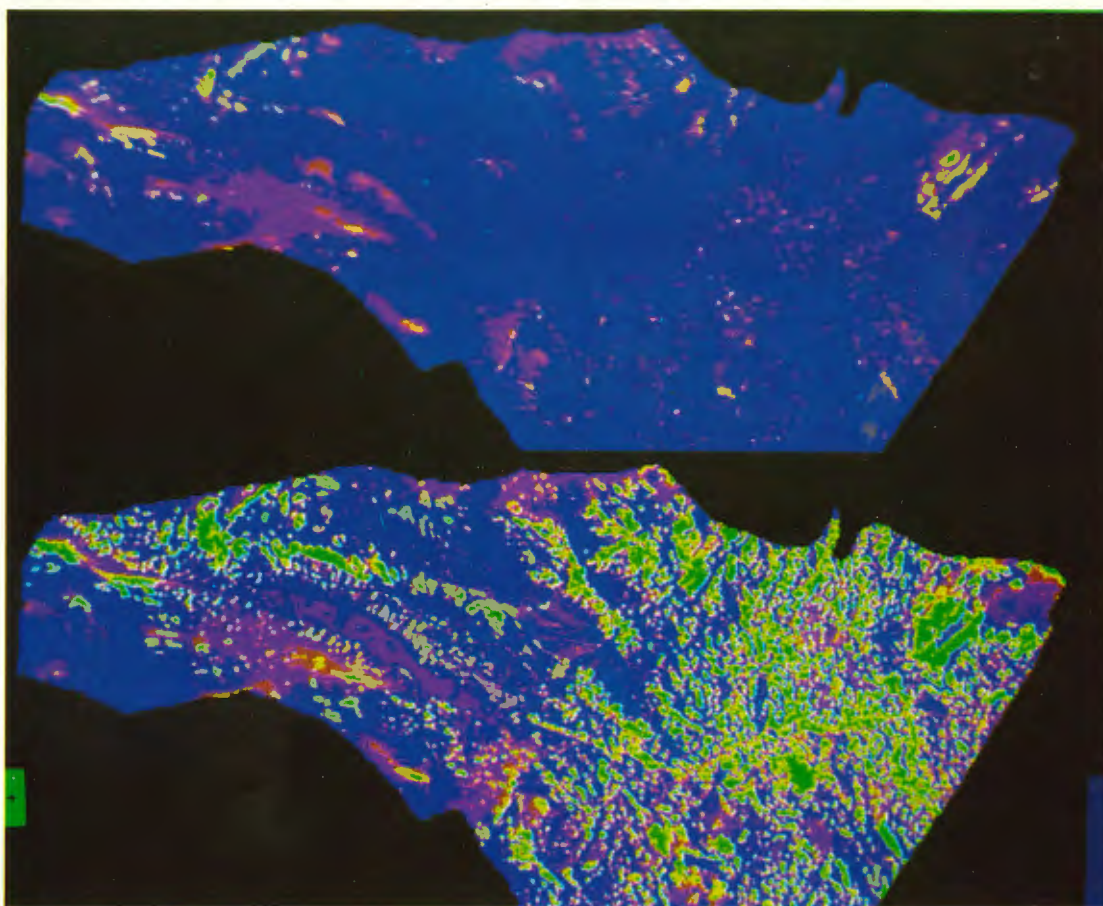
Figur 3. Den beräknade snötäckningsgraden fördelad på klasser för den 25 maj (överst) och den 6 juni. Grönt innebär 0 - 20 % snötäckningsgrad, gult 20 - 40 %, ljusviolettt 40 - 60 %, mörkviolettt 60 - 80 % och blått 80 - 100 %.
