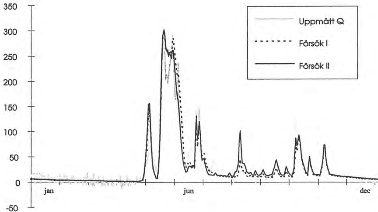
Figur 10: Resultat av simulering med standard HBV-modellen (Försök I) och avdunstningens höjdberoende inlagt explicit i modellen (Försök II) för Torröns avrinningsområde år 1984.
