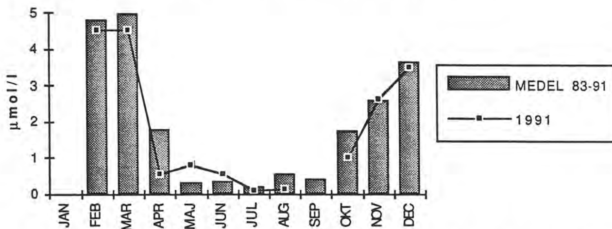
F64b NO3-N 10 meters djup 1991 och medel 1983-91
