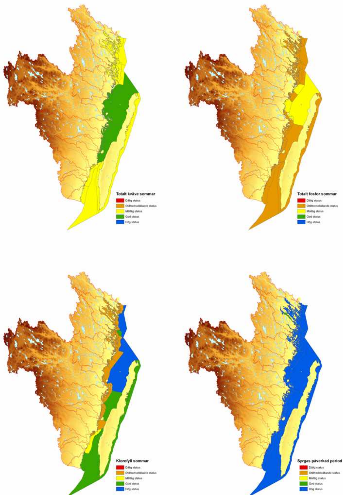
Figur 8. Smålandskusten . Statusklassificering beräknat med hjälp av HOME Vatten för perioden 2001-2005. Klassificeringen avser sommarvärden i ytan för total-kväve, total-fosfor och klorofyll, dvs. integrerade värden för de 10 översta metrarna under juni - augusti. Klassificeringen för syrgas avser bottenvattnet för den påverkade perioden (juni-december). Klasserna baseras på typindelningen av svenska övergångs- och kustvatten enligt Ramdirektivet för Vatten. Färgskalan på land indikerar höjd över havet.
