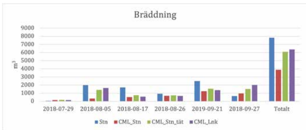
Figur 8. Beräknad bräddmängd (m³) vid olika regntillfällen utifrån olika regndataset.
