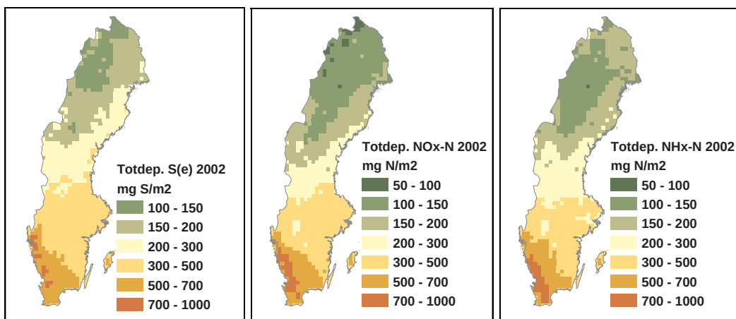
Figur 11. Total deposition (våt+torr) av svavel (exklusive havssalt), NO x -kväve och NH x -kväve för år 2002.
