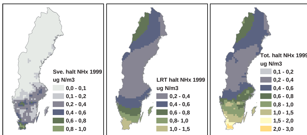
Figur 4. Årshalt av NH x -kväve i luft uppdelat på Sveriges bidrag, långtransporterat bidrag och totalt för år 1999.
