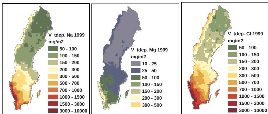
Figur 3. Våtdeposition av natrium (Na), magnesium (Mg) och klor (Cl) för år 1999.
