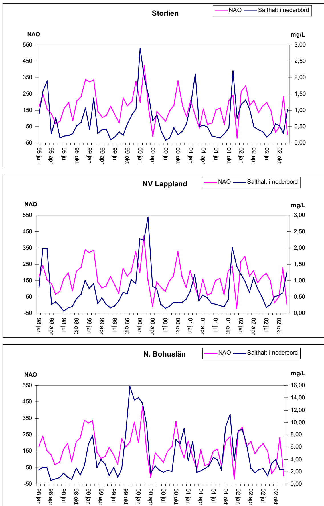
Figur 14. Månadsvärden för perioden 1998-2002 av NAO-index jämfört med havssaltkoncentration (mg klorid/L) i nederbörd för tre områden i västligaste Sverige (norra Bohuslän, nordvästra Lappland och västligaste Jämtland).
