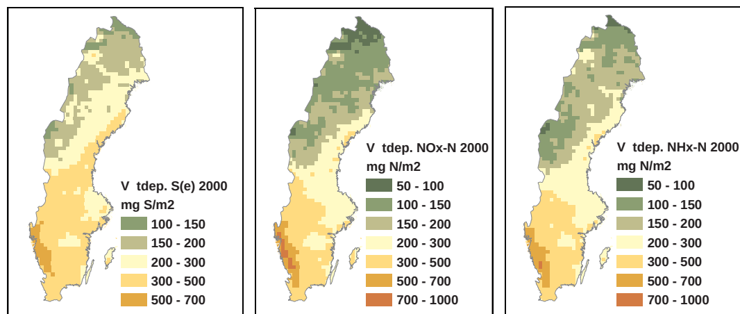
Figur 6. Våtdeposition av svavel (exklusive havssalt), NO x -kväve och NH x - kväve för år 2000.
