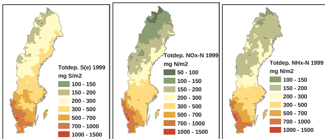
Figur 2. Total deposition (våt+torr) av svavel (exklusive havssalt), NO x -kväve och NH x -kväve för år 1999.
