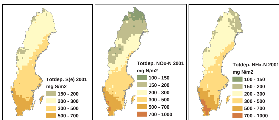
Figur 8. Total deposition (våt+torr) av svavel (exklusive havssalt), NO x -kväve och NH x -kväve för år 2001.
