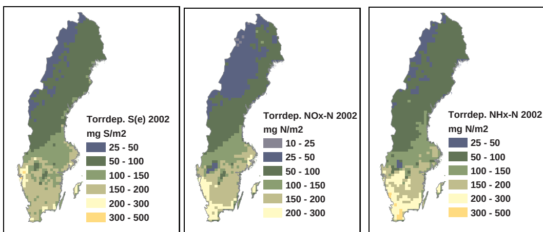
Figur 12. Torrdeposition av svavel (exklusive havssalt), NO x -kväve och NH x -kväve för år 2002.
