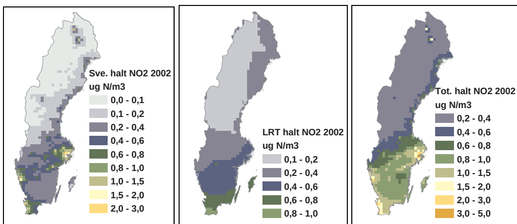
Figur 13. Årshalt av NO 2 i luft uppdelat på Sveriges bidrag, långtransporterat bidrag och totalt för år 2002.
