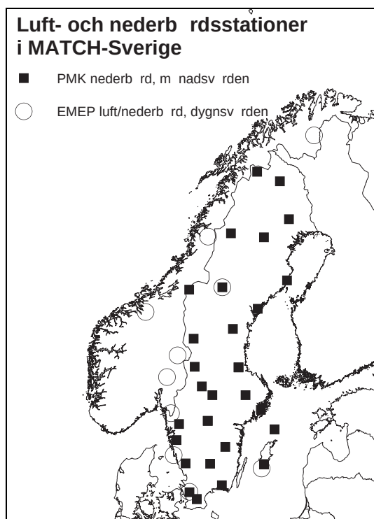
Figur 1. Atmosfärkemiska bakgrundsstationer som utnyttjats för MATCH-Sverige beräkningarna.
