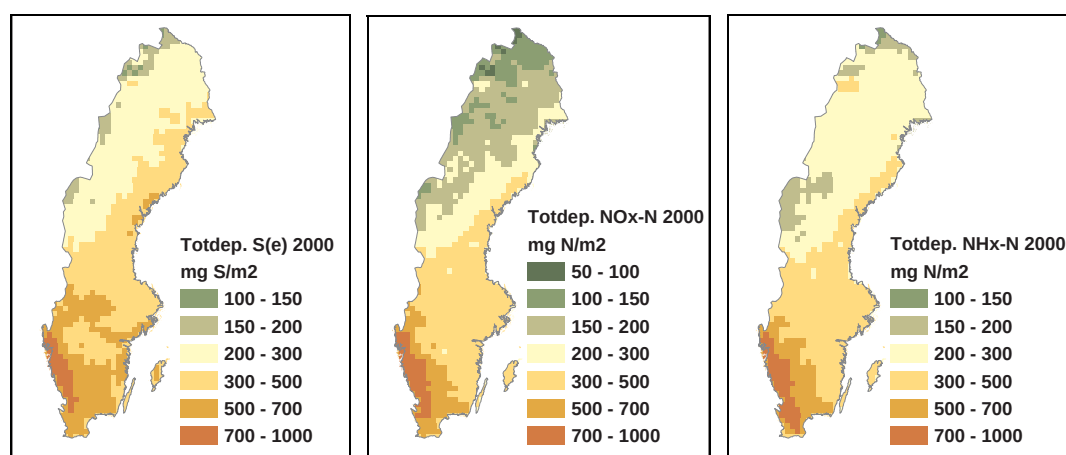
Figur 5. Total deposition (våt+torr) av svavel (exklusive havssalt), NO x -kväve och NH x - kväve för år 2000.
