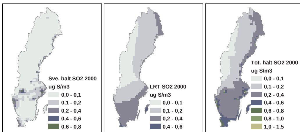
Figur 7. Årshalt av SO 2 i luft uppdelat på Sveriges bidrag, långtransporterat bidrag och totalt för år 2000.
