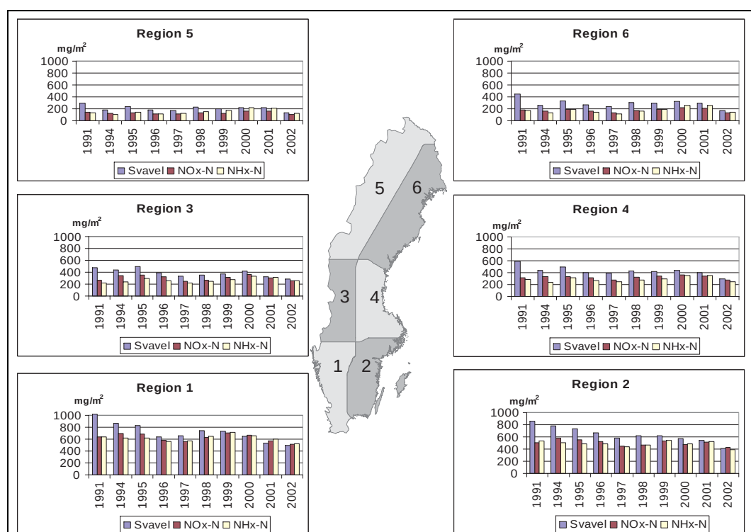
Figur 15. Trender för åren 1991, 1994-2002 utförda för sex regioner i Sverige. Modellresultaten för de olika åren baseras på olika modellversioner, och resultaten måste därför ses som preliminära.
