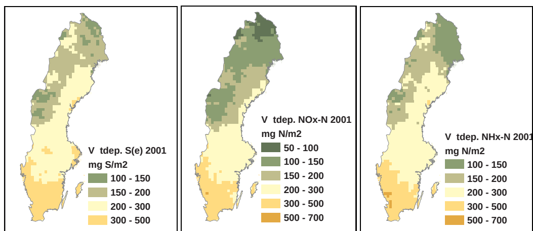
Figur 9. Våtdeposition av svavel (exklusive havssalt), NO x -kväve och NH x -kväve för år 2001.
