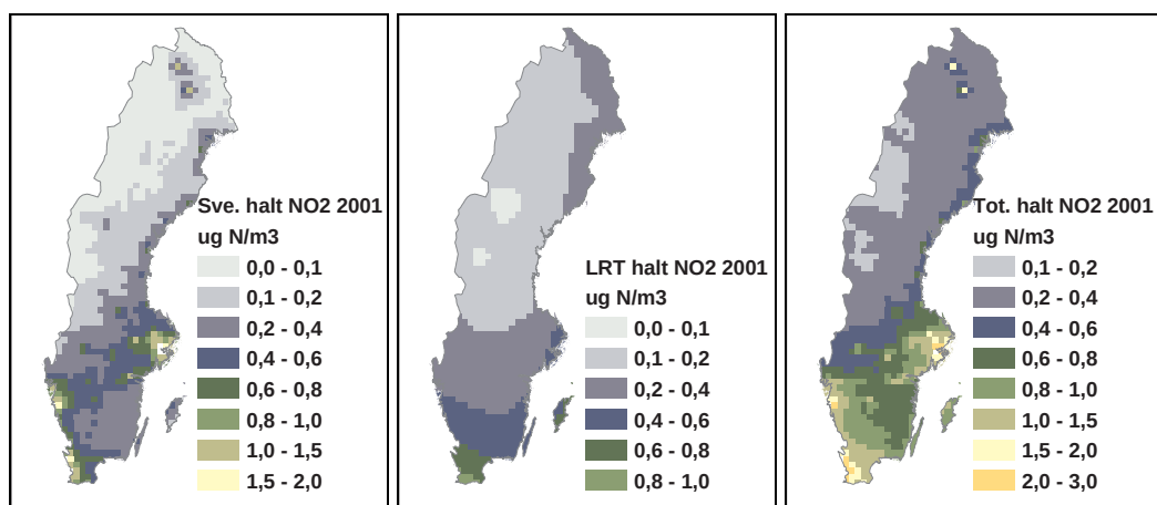
Figur 10. Årshalt av NO 2 -kväve i luft uppdelat på Sveriges bidrag, långtransporterat bidrag och totalt för år 2001.
