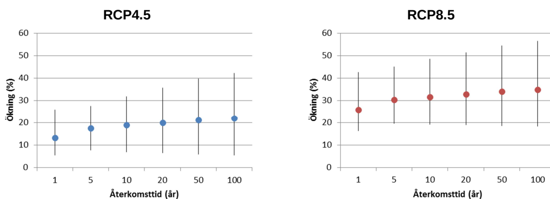
Figur 4. Procentuell förändring av nederbörd med varaktigheten 1 timme mellan perioderna 2069-2098 och 1961-1990 för Södermanlands län. Punkterna representerar medianvärden och vertikala streck visar spridningen mellan de olika modellberäkningarna.
