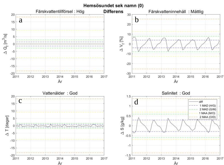
Figur 37. Svart kurva visar differensen (ekvation 3) mellan den normala och den naturliga tidsserien för delparametrarna i Hemsöundet. Klassgränserna H/G (blå linjer), G/M (gröna linjer), M/O (gula linjer) och O/D (orange linjer) är specifika för kustvattenförekomsten.
