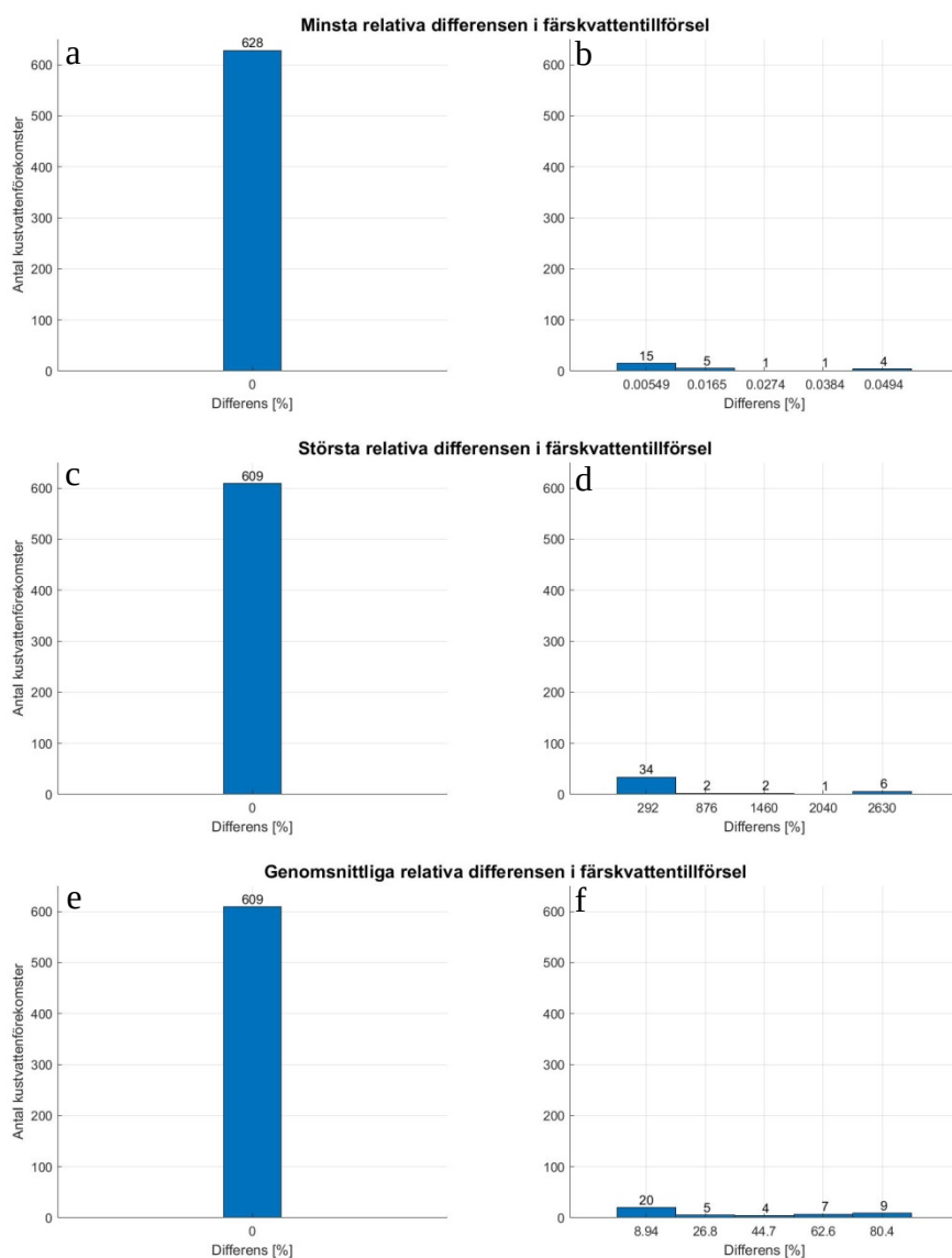
Figur 9. Fördelning av minsta relativa, största relativa och genomsnittliga relativa differens i färskvattentillförsel beräknat enligt ekvation 2.
