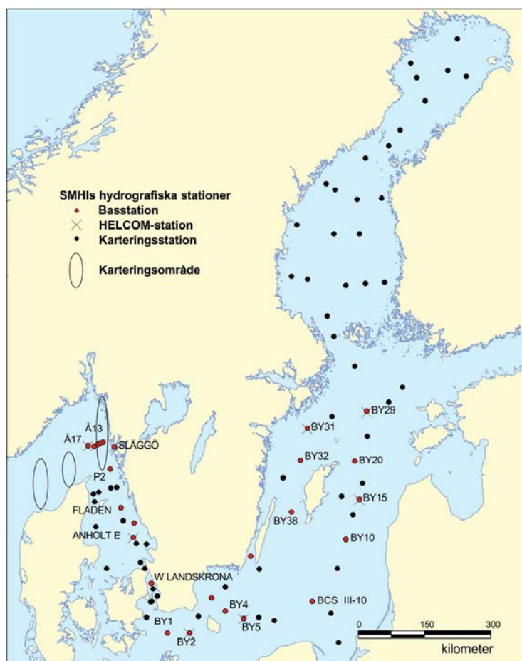
Figur 1. De rödmarkerade basstationerna provtas 12 ggr/år. Undantag: BY31 och BY29 provtas endast 4 ggr/år (vintertid) av SMHI.
