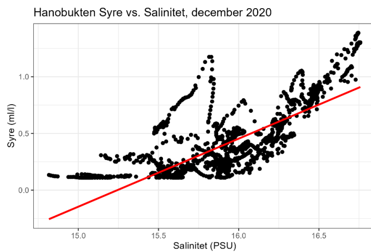
Figur 11. Visuell korrelationsanalys mellan salinitet och syre för perioden december 2020 – oktober 2021 (A-B), och mellan salinitet och syre för perioden december 2020 (C). Observationer för olika månader indikeras med specifika färger. Röd linje indikerar resultatet av en linjär regressionsanalys.
