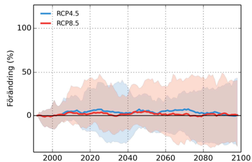
Köpingsåns mynning
