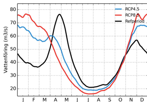
Hedströmmens mynning
