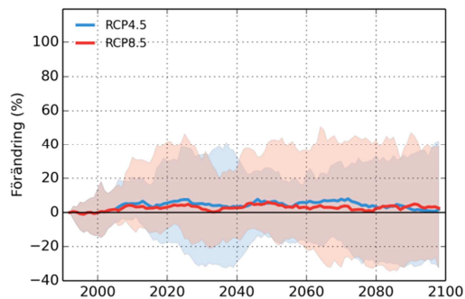
Hedströmmens mynning
