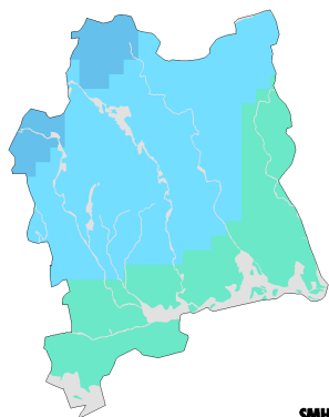
Beräknat 2021-2050
