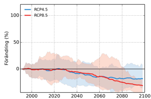
Kolbäcksåns mynning
