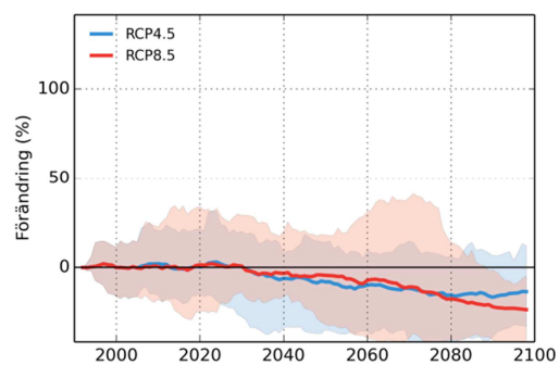
Sagåns mynning
