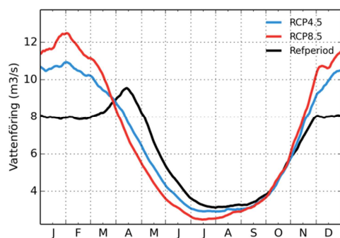
Svartåns mynning
