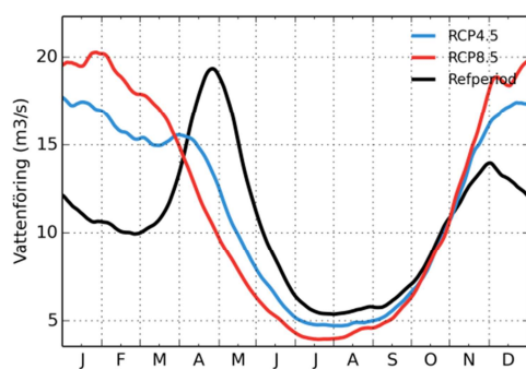
Kolbäcksåns mynning
