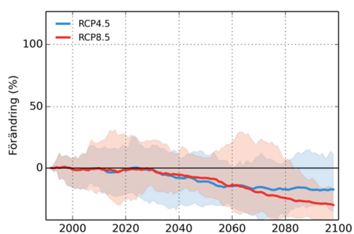
Köpingsåns mynning
