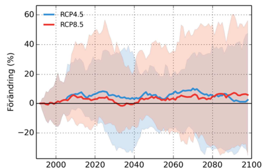
Sagåns mynning
