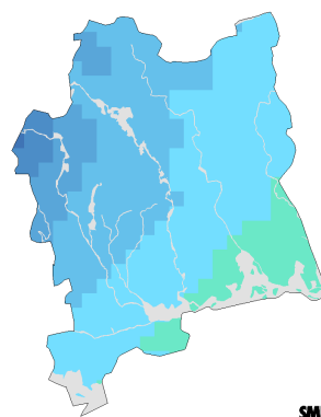
Beräknat 2069-2098
