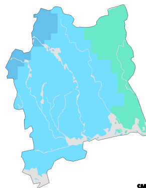
Beräknat 2069-2098
