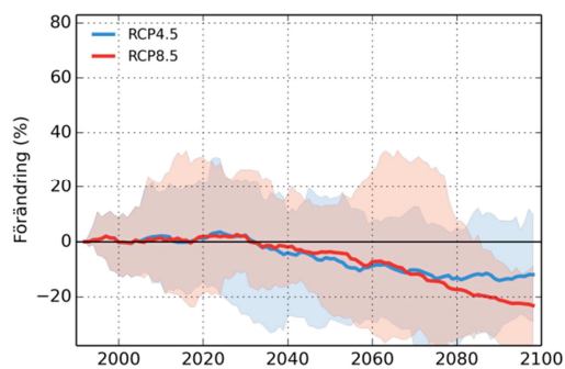
Svartåns mynning
