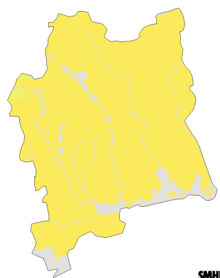
Beräknat 2069-2098
