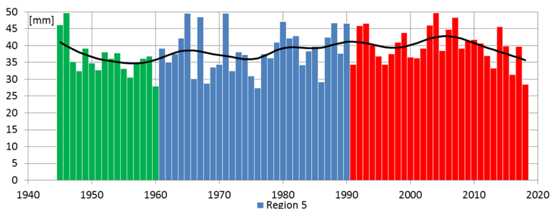
Figur 32 Medelvärde av årshögsta punktnederbörden över 24 timmar perioden 1945-2018 för var och en av de 5 regionerna i riktlinjerna. Den svarta linjen representerar ett flytande 10-årsmedelvärde framtaget med ett Gauss-filter.
