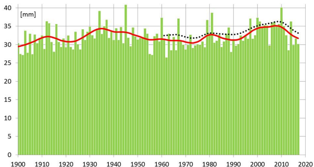
Figur 33 Medelvärde av årets största dygnsnederbörd (staplar) som bygger på 60 utvalda stationer i hela Sverige. Röd kurva visar en utjämnad kurva av staplarna. Prickad svart kurva visar en utjämnad kurva av samtliga stationer som varit i drift under året.
